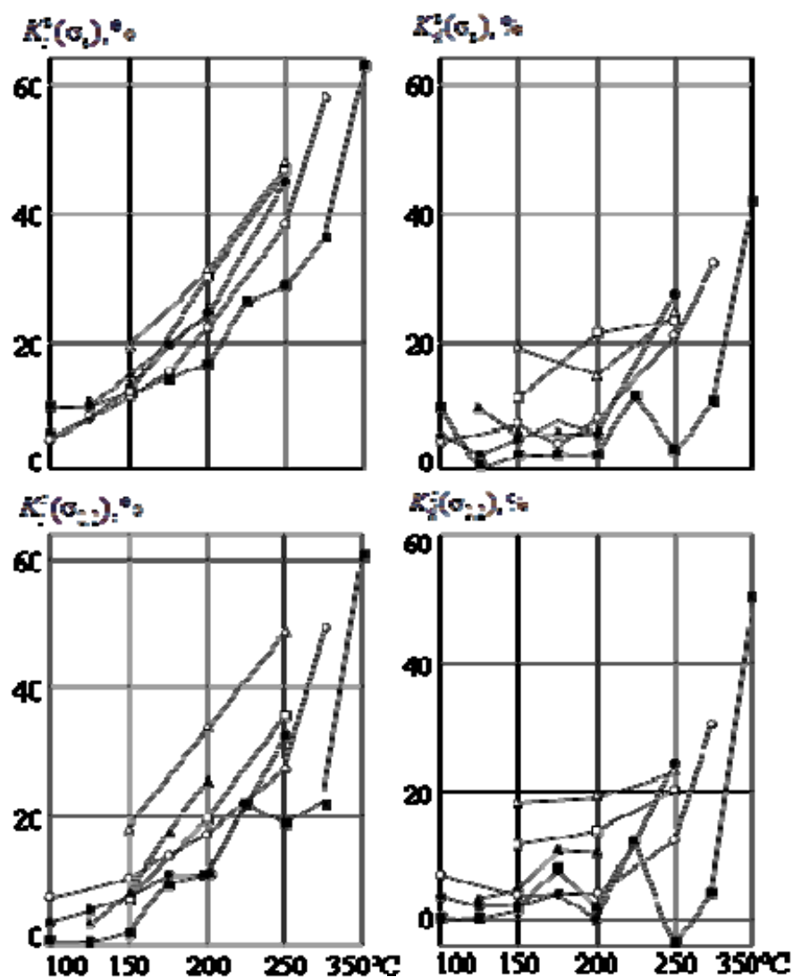
Рис. 3. Характер изменения темпа разупрочнения ( K_i^B ; K_d^B ; K_i^S ; K_d^S ) при температуре 100-350°C жаропрочных конструкционных алюминиевых сплавов систем Al-Cu-Mg и Al-Cu (плакированный (А) лист толщиной 2-3 мм, направление: П, кратковременные испытания, статическое растяжение):
