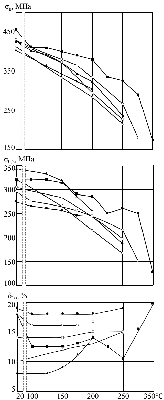
Рис. 2. Характер изменения значений механических свойств при 100-350°C плакированных листов толщиной 2-3 мм жаропрочных конструкционных алюминиевых сплавов (направление: П) систем Al-Cu-Mg и Al-Cu (кратковременные испытания, статическое растяжение): 1151-T (■); Д19-T (○); Д16-T (●); АК4-1ч.-T1 (T2) (▲); Д21-T1 (□); 1201-T1 (Δ)
